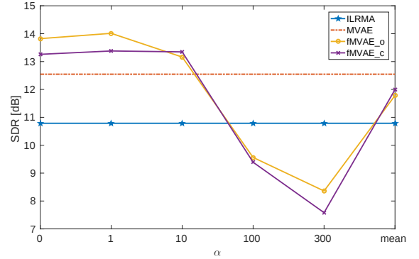
図 2: 話者依存条件での \alpha の設定値による SDR 平均値 [dB] の違い.
