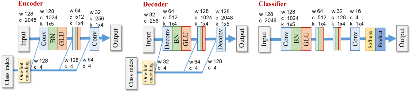
図 1: ACVAE のネットワーク構造. 入力と出力スペクトログラムの周波数軸をチャネル軸と見なし, 1 次元畳み込み NN を用いる. “w”, “c” と “k” はそれぞれデータの系列長, チャネル数とフィルタサイズを表し, “Conv”, “Deconv”, “BN” と “GLU” はそれぞれ畳み込み, 逆畳み込み, バッチ正規化と gated linear unit と呼ばれるデータ駆動の活性化関数を表す.
