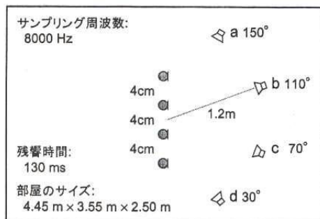
図 2: 部屋の特性とスピーカ/マイクの配置
