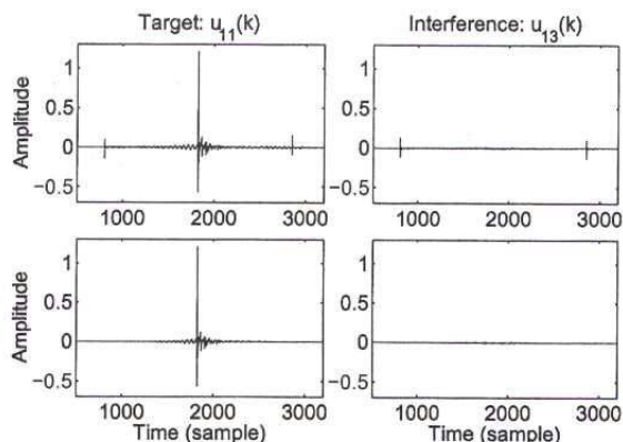
図 3: 3 音源分離における離散周波数表現の巡回性による影響 (上段) と smoothing の効果 (下段)
