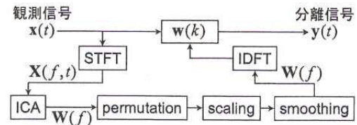
図 1: 周波数領域 BSS の処理の流れ
