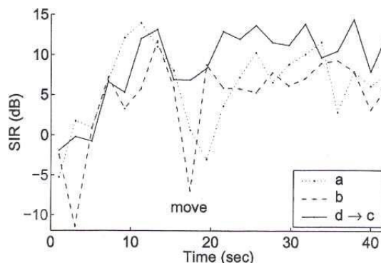
図 4: 音源移動に対するリアルタイム処理の分離性能
